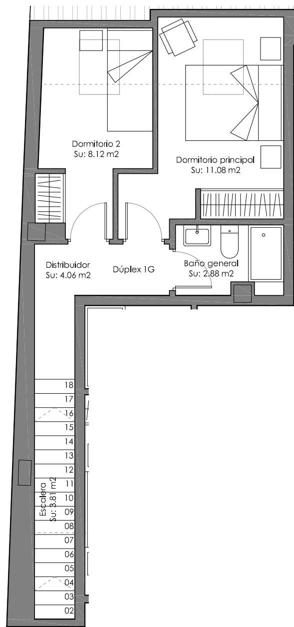
PLANTA SEGUNDA, PISO 1º G - USOS Y SUPERFICIES e. 1/75
