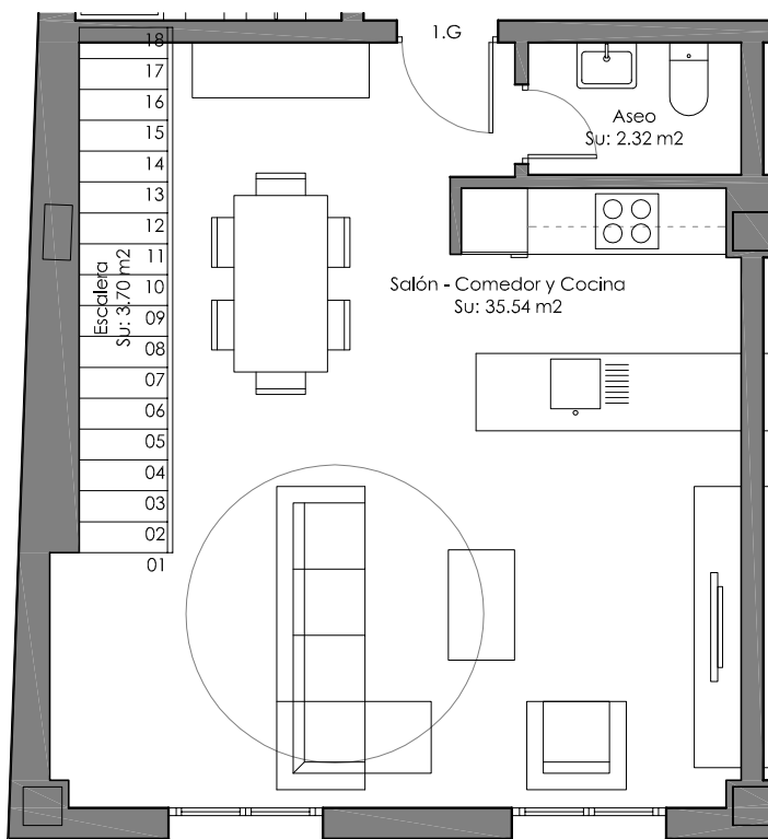
PLANTA PRIMERA, PISO 1º G - USOS Y SUPERFICIES e. 1/75
