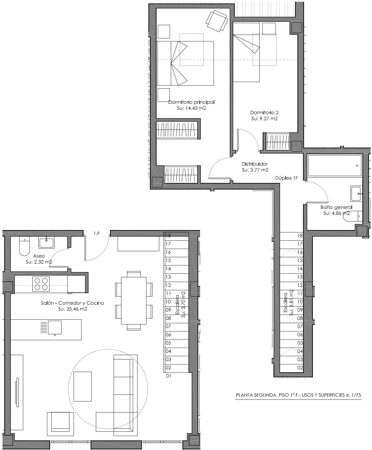
PLANTA PRIMERA, PISO 1º F - USOS Y SUPERFICIES e. 1/75
