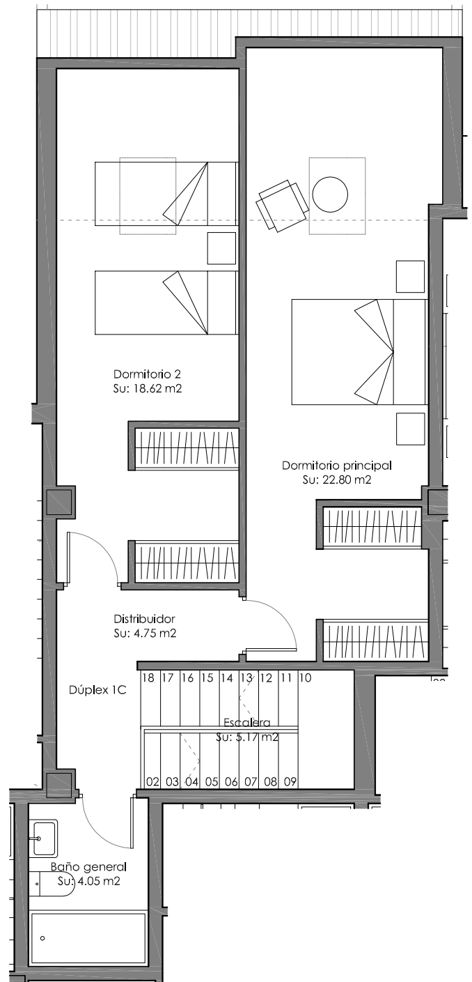
PLANTA SEGUNDA, PISO 1º C - USOS Y SUPERFICIES e. 1/75
