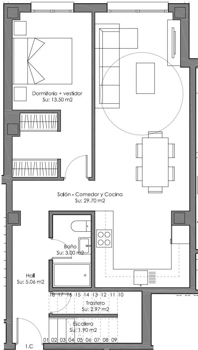
PLANTA PRIMERA, PISO 1º C - USOS Y SUPERFICIES e. 1/75
