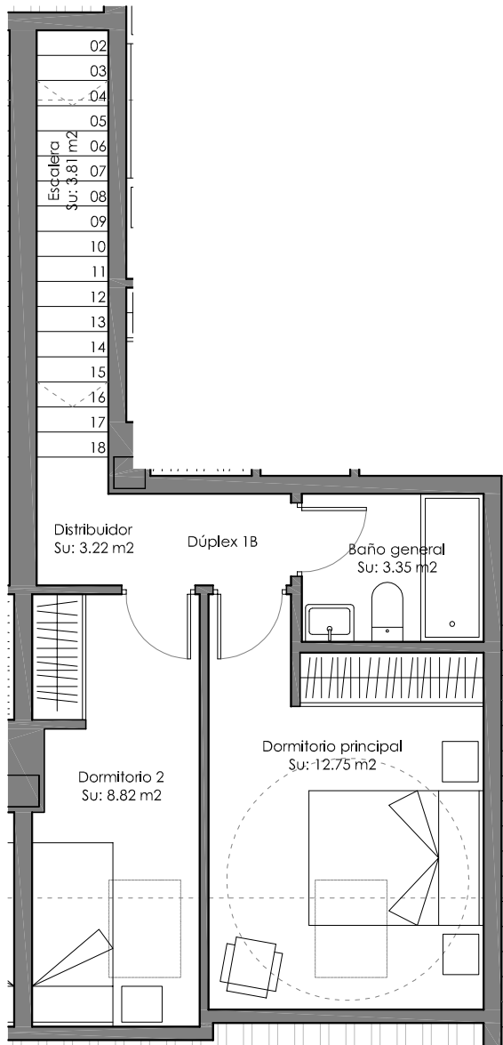
PLANTA SEGUNDA, PISO 1º B - USOS Y SUPERFICIES e. 1/75
