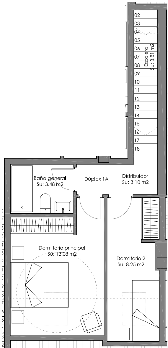
PLANTA SEGUNDA, PISO 1º A - USOS Y SUPERFICIES e. 1/75
