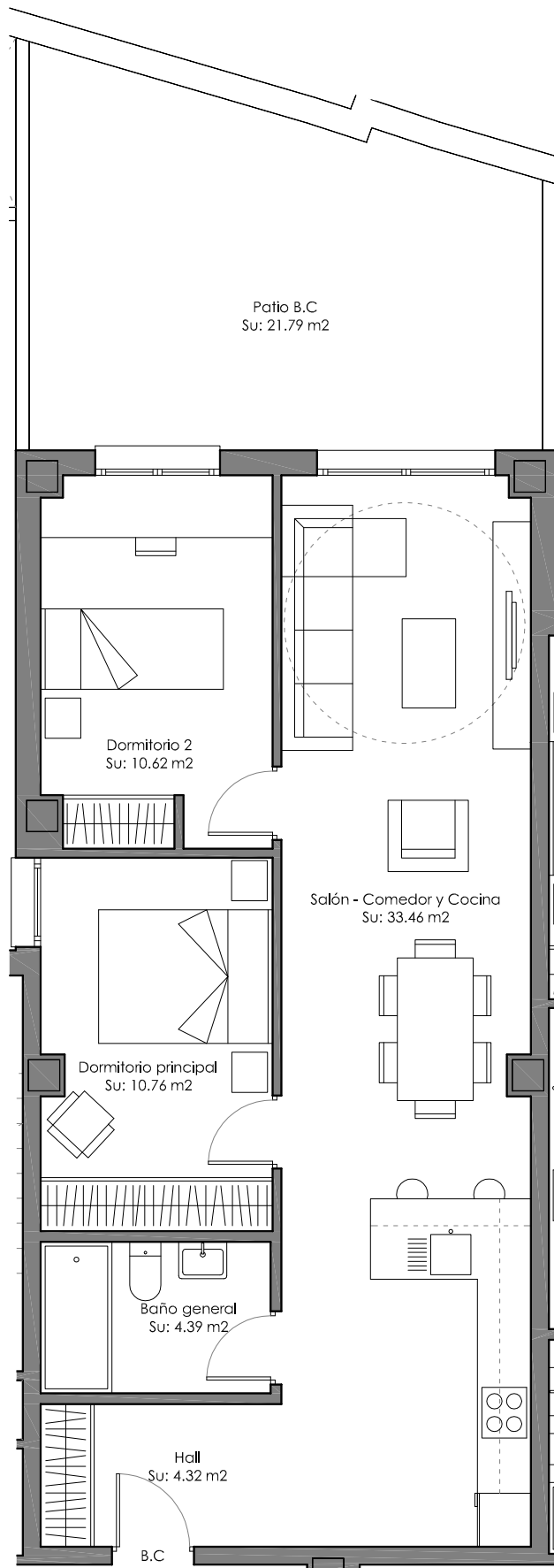
PLANTA BAJA, PISO B° C - USOS Y SUPERFICIES e. 1/75
