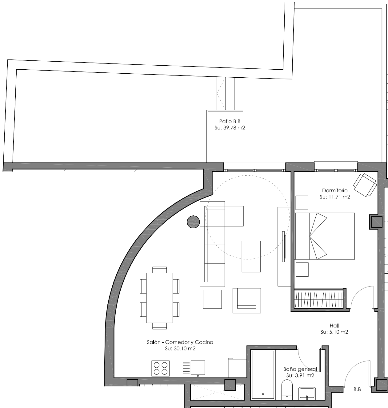
PLANTA BAJA, PISO Bº B - USOS Y SUPERFICIES e. 1/75
