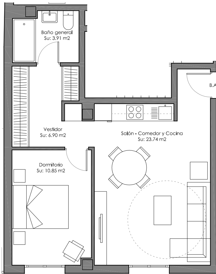
PLANTA BAJA, PISO Bº A - USOS Y SUPERFICIES e. 1/75
