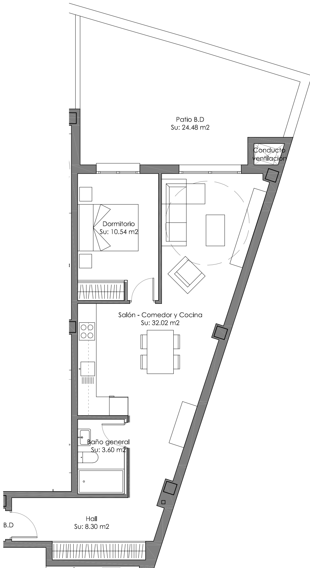
PLANTA BAJA, PISO Bº D - USOS Y SUPERFICIES e. 1/75
