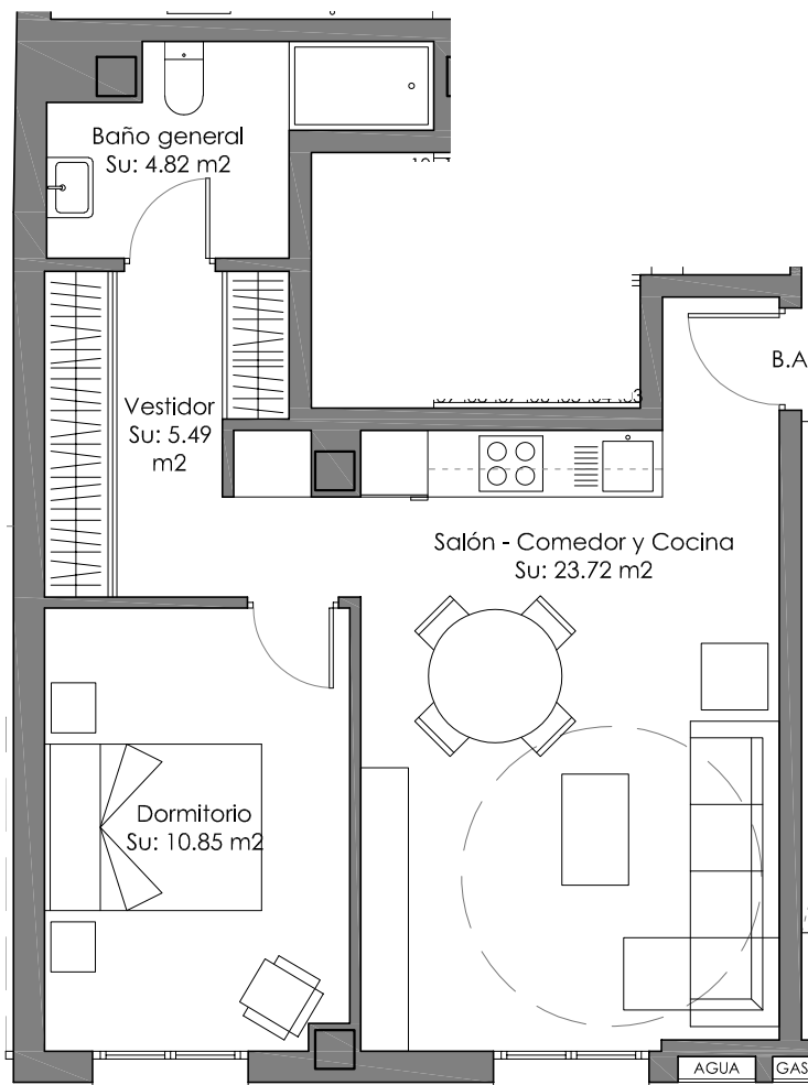
PLANTA BAJA, PISO Bº A - USOS Y SUPERFICIES e. 1/75
